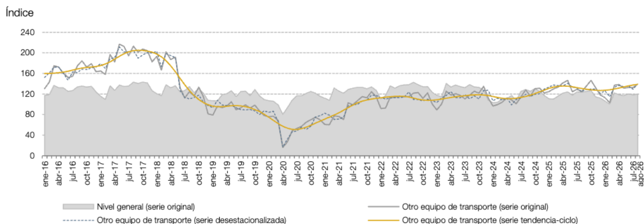
Gráfico 2.15.a Otro equipo de transporte con respecto al nivel general de la serie original del IPI manufacturero. Enero 2016-agosto 2026
