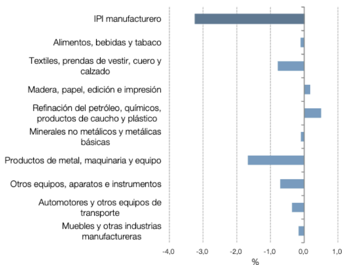
Gráfico 1.3 IPI manufacturero nivel general y categorías, incidencias. Agosto de 2026*
