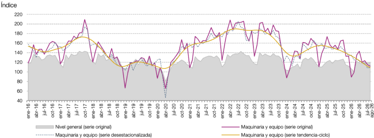
Gráfico 2.12.a Maquinaria y equipo con respecto al nivel general de la serie original del IPI manufacturero. Enero 2016-agosto 2026
