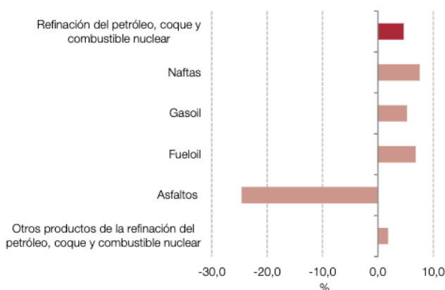
Gráfico 2.6.b Refinación del petróleo, coque y combustible nuclear, variación porcentual interanual. Agosto de 2026*
